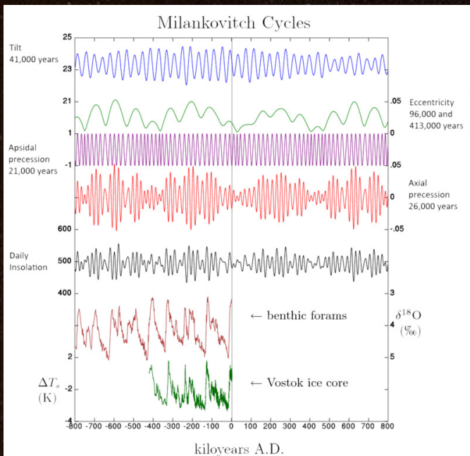
Resim: Milankovitch Döngüleri.
