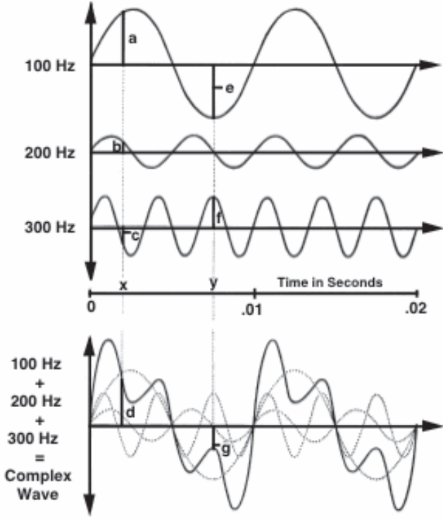
Resim: Fourier Analizi.
